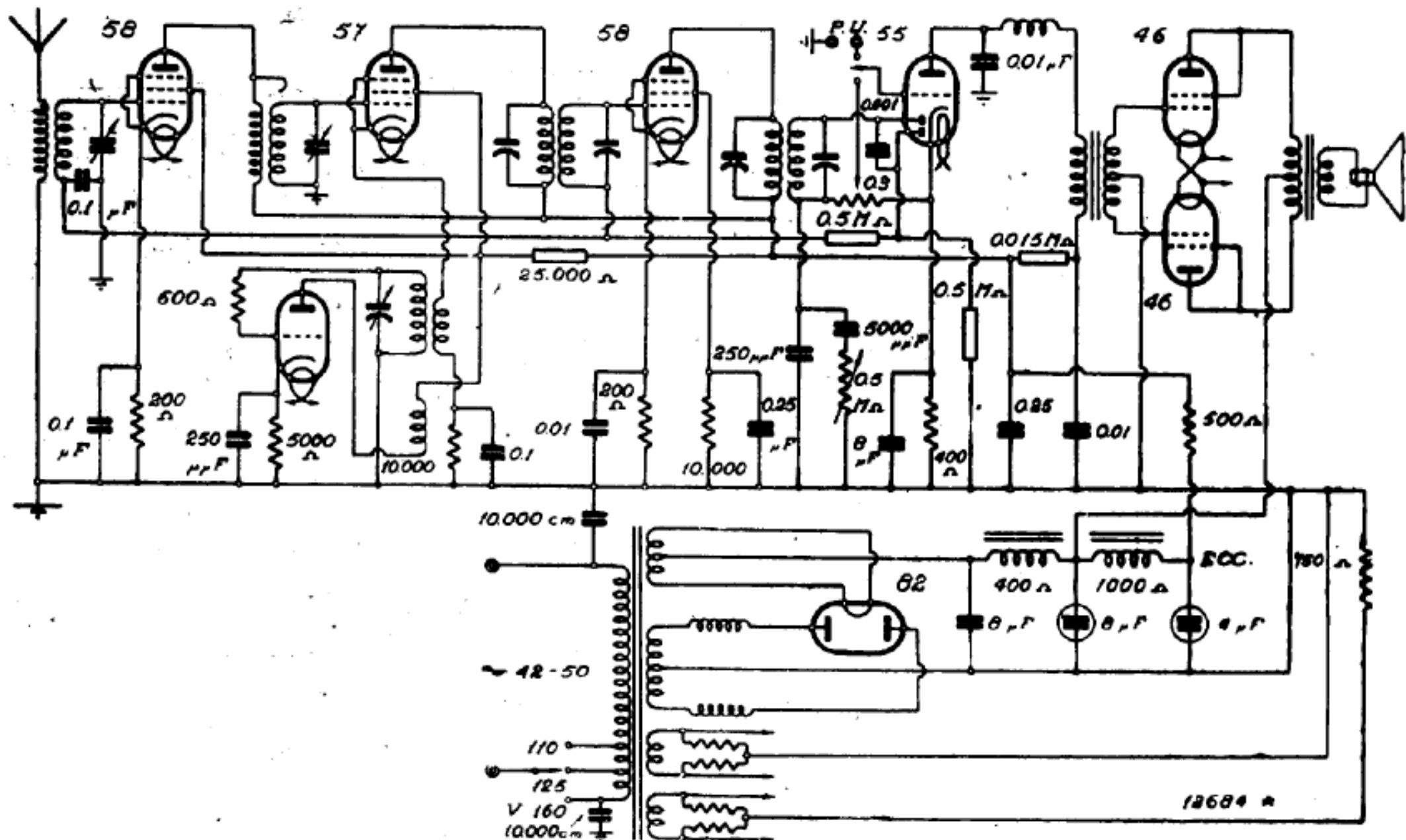
CRESA RADIO - MOD. « SUPERLA 8 CA »
